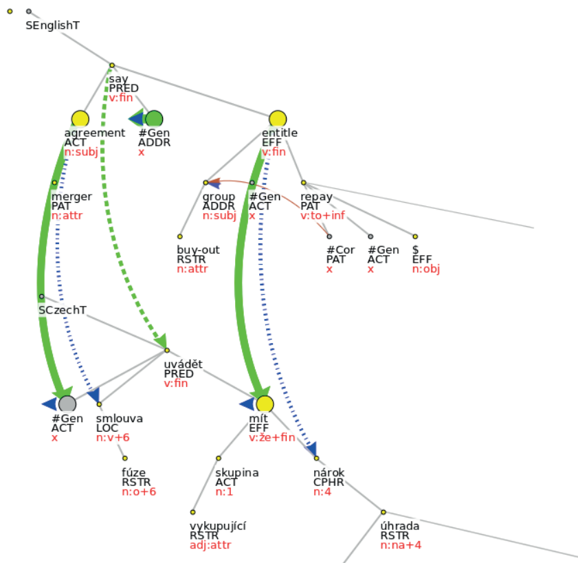
OBR. 2 — Část tektogramatického stromu ukazující konflikt slovníkového a reálného mapování participantů. Zelené šipky ukazují nepříznačné uložené slovníkové mapování (ACT- ACT ), modré šipky navržené mapování faktické (ACT- LOC ).
