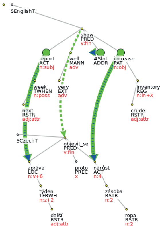
OBR. 1 — Functor mismatch. Mapování participantů větné struktury pro dvojici vět:
